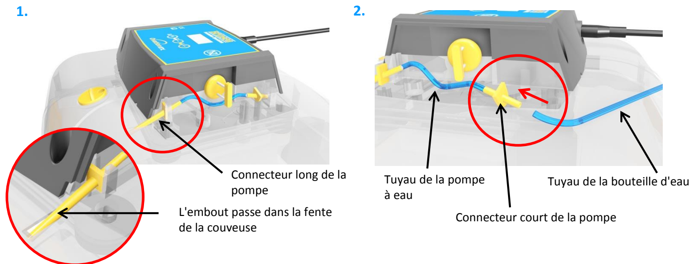
Diagramme du tuyau à l'échelle
